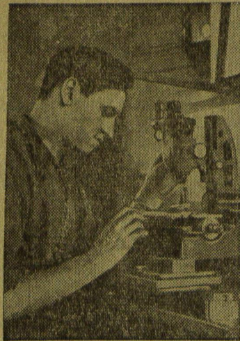
ЛЕНИНГРАД. Слесарь-кальщик завода «Электросила» имени С. М. Кирова коммунист В. И. Мейель за 2 года 7 месяцев выполнил одиннадцать годовых норм. На снимке: В. И. Мейель промеряет деталь инструментальным микроскопом.
